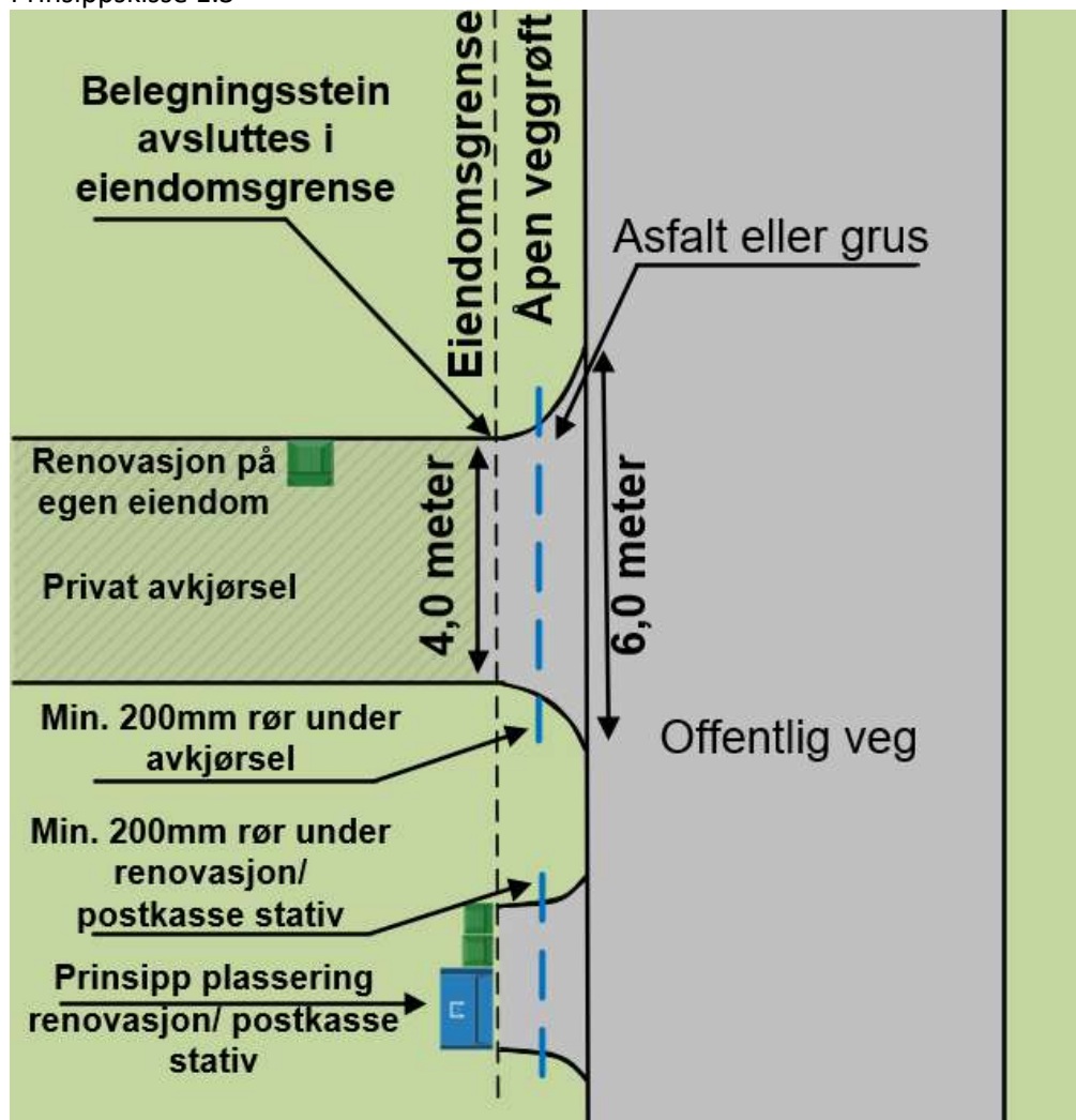
Prinsippskisse 1.3
