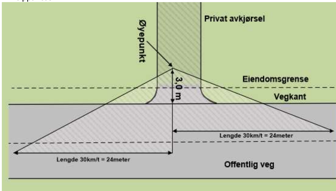
Prinsippskisse 1.1
